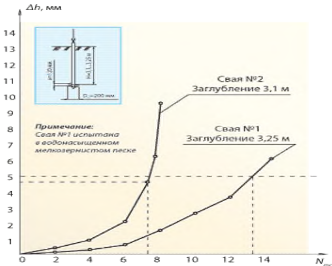
Рис. 1. График испытания свай на выдергивание в водонасыщенном песке.
